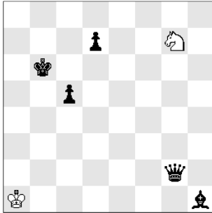
h#6,5 (2+5)
