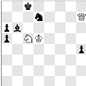
s#7 Längstzüger (3+6)
