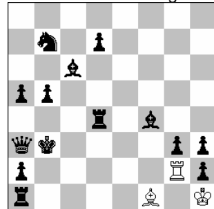
h#3 b) sDa3->b4 (3+14)
